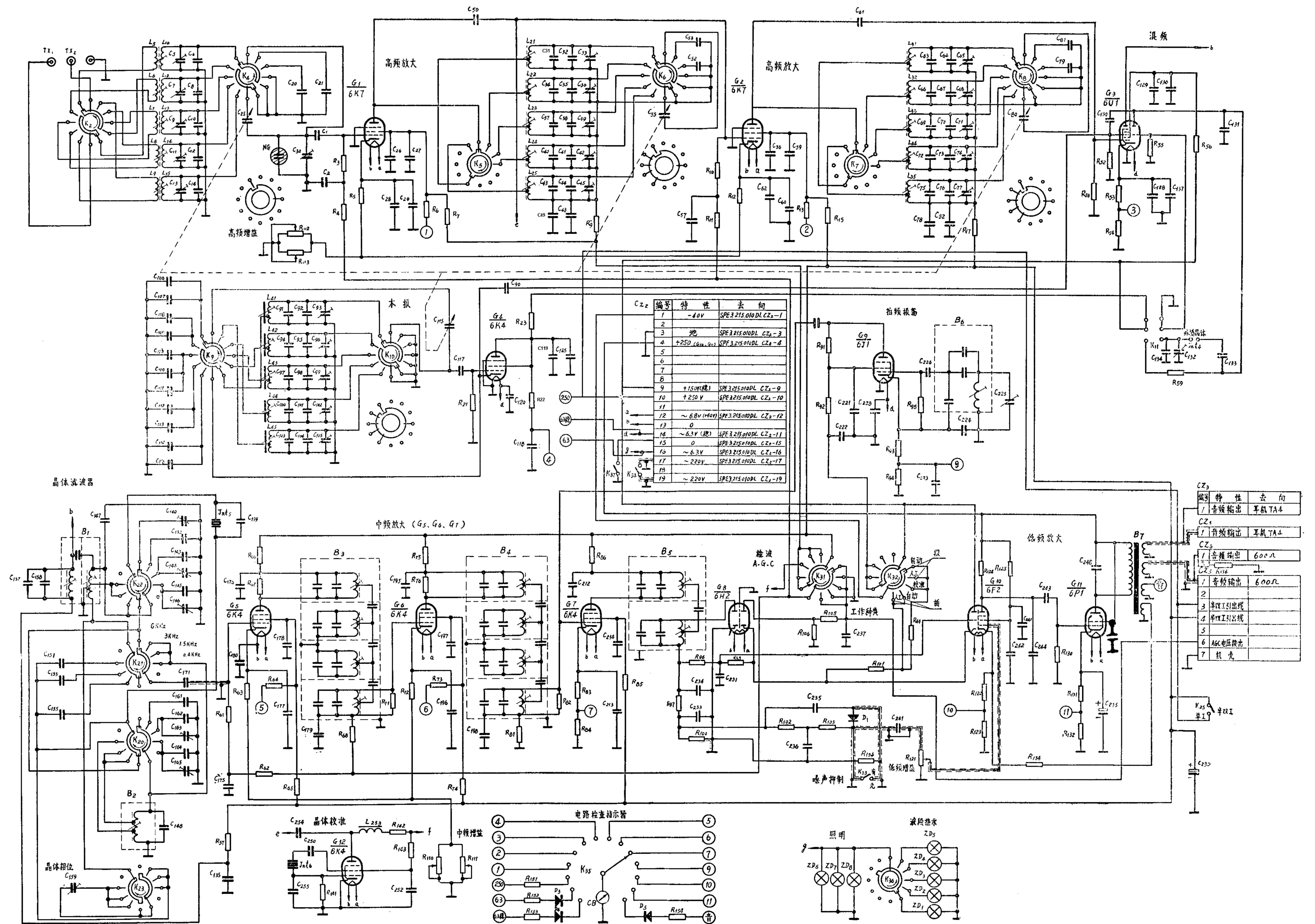
5. 收音机电原理图
